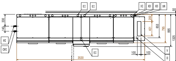
Boven aanzicht
